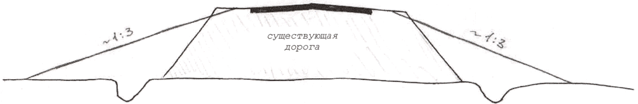
Вариант 2 Устройство откосов уклоном 1:3 \dots 1:4
