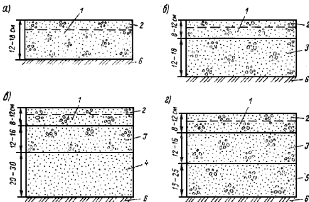
Рис. 1.2. Примеры конструкций дорожных одежд с гравийными покрытиями:
