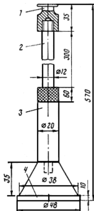
Рис. 2. Уплотнитель:
