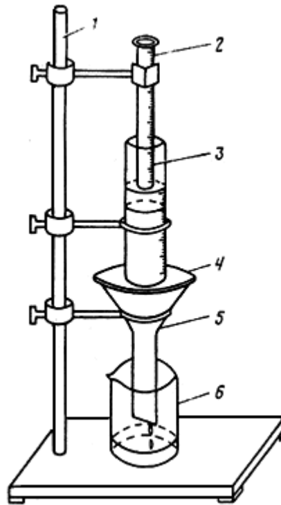
Рис. 1. Прибор для определения водостойкости лигносульфонатов технических
