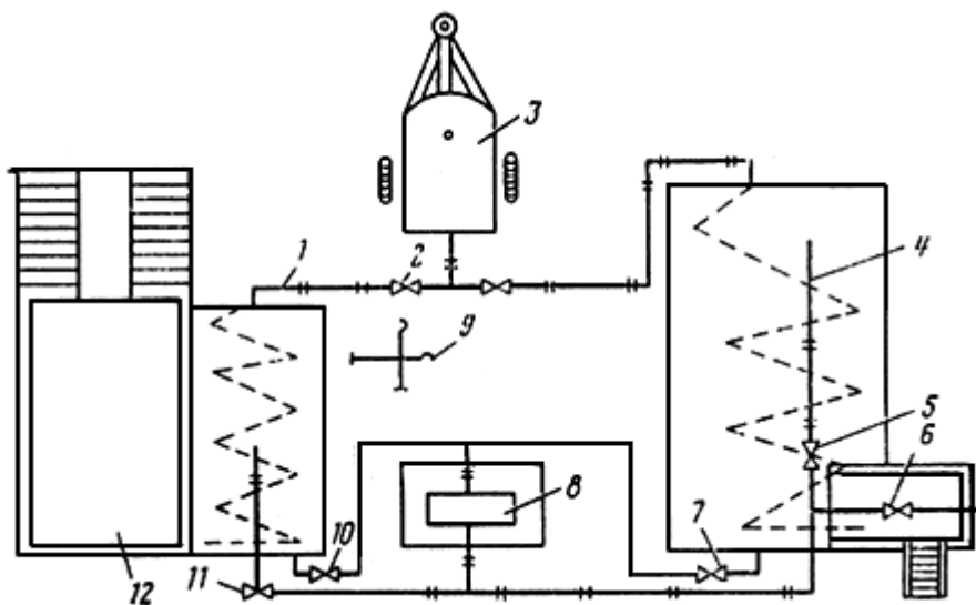
Рис. 1. Схема установки для приготовления обеспыливающих растворов
