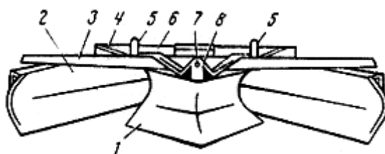
Рис. 3.2. Плужный смеситель:
