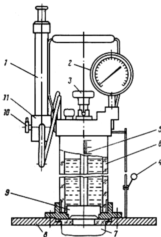
Рис. 1. Общий вид прибора КП-120
